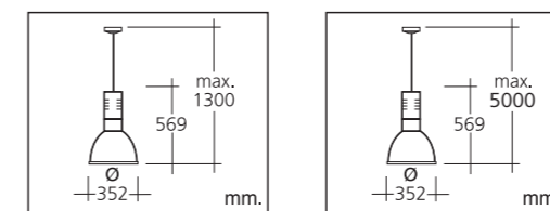
mit 3-Phase Multi Adapter
